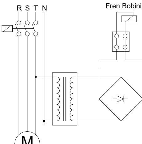
Gecikmeli Frenleme / Delayed Running Brake / Verspätete Bremsung ( 24 V )
